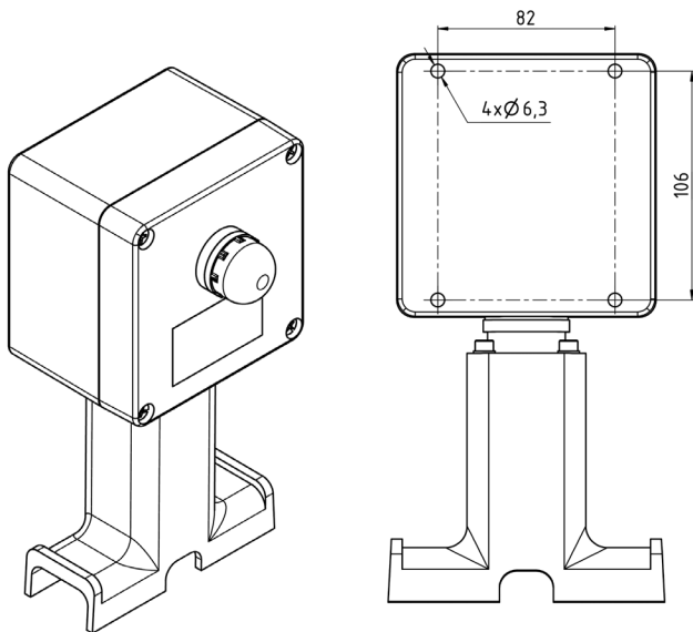
Установочные размеры
